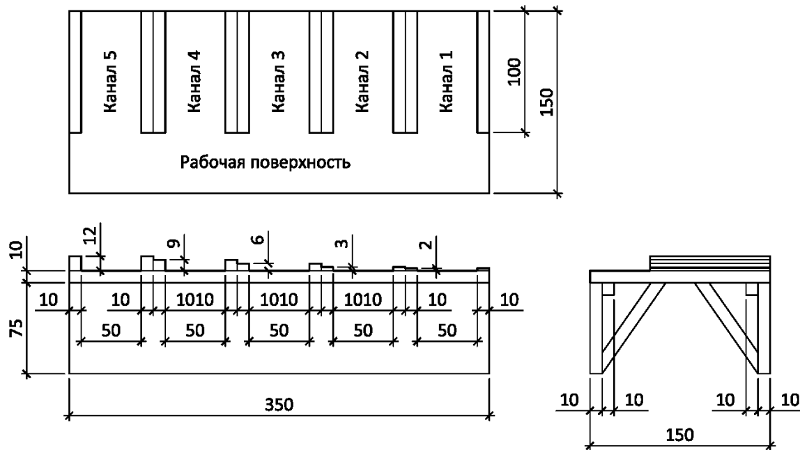
Рисунок Б.1 – Стенд испытательный стальной
