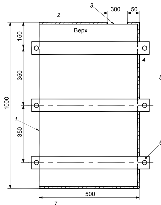
Рисунок Д.1 – Форма и размеры сборного образца-плиты
