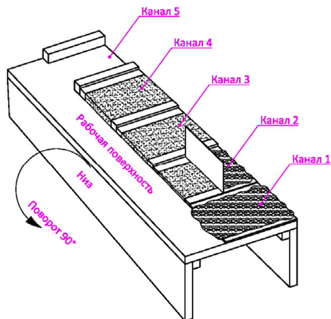
Рисунок Б.1 – Стенд испытательный стальной
